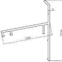
8 - PROFILO DI COPIERTURA DELLA PARETE
