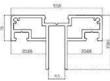
5 - PROFILO COPERTURA SUPPORTO IN VETRO
