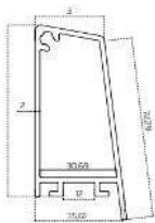
2 - ESTENSIONE PROFILO GRONDAIA
