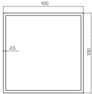
3 - PROFILO SCATOLA
